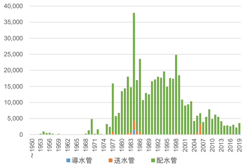
図表 2-20 上水道管渠の建設年度と延長距離
