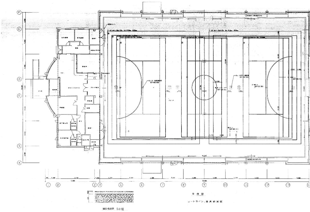
市営多目的屋内運動場平面図
