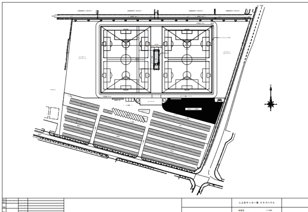
巾宮人工芝サッカーフィールド平面図
