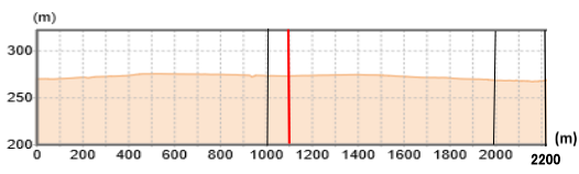
第2区縦断面図 興譲館高校西～佐藤 了車庫前 2.220Km
