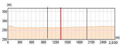
第3区縦断面図 佐藤 了車庫前～窪倉公民館前 2.630Km
