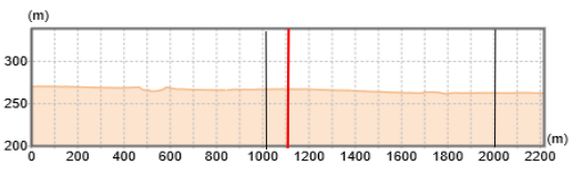
第4区縦断面図 窪倉公民館前～競技場 2.220Km
