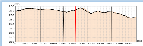
第4区 縦断面図
