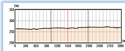
第2区 縦断面図
