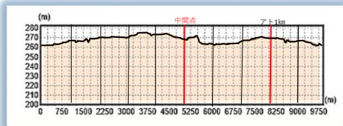
第1区 縦断面図
