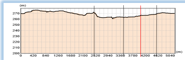
第3区 縦断面図
