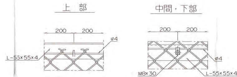
金網取付詳細図 S=1/4
