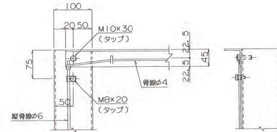
A'部詳細図 s=1/5
