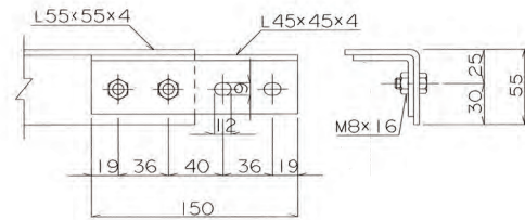
胴縁継手部 s=1/3
