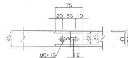
胴縁継手部 s=1/3
