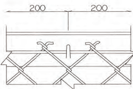
金網取付部 s=1/3
