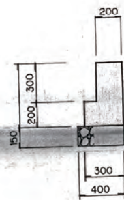
A-A 断面 S=1:20
