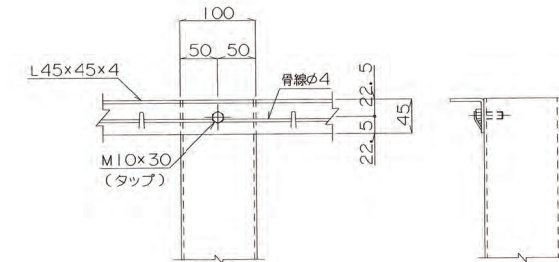
A部詳細図 s=1/5
