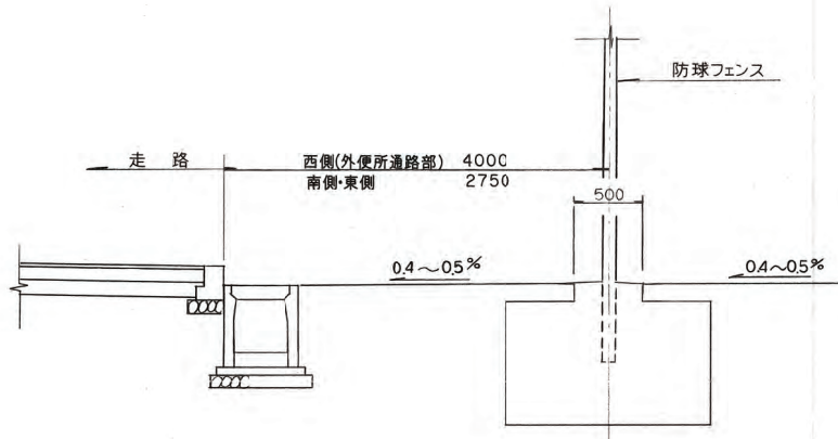
防球フェンス配置断面図 S=1:30
