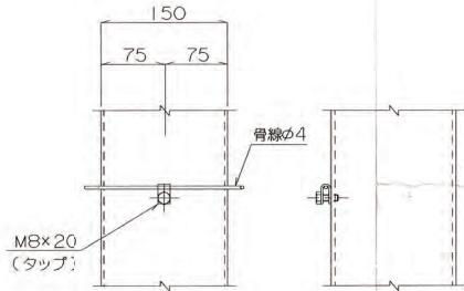
C部詳細図 s=1/5
