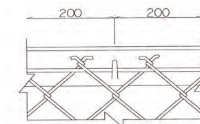
金網取付部 s=1/3
