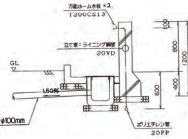
足洗場断面詳細図 S=1:30
