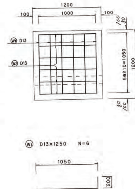
壁配筋図
