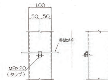
B部詳細図 s=1/5
