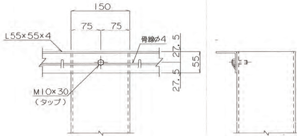
A部詳細図 s=1/5
