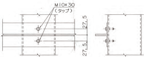
B部詳細図 s=1/5
