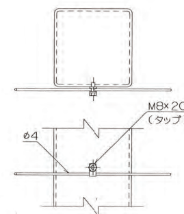
D部詳細図 S=1/6
