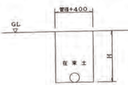
排水管地中埋設要領図 NO. SCALE
