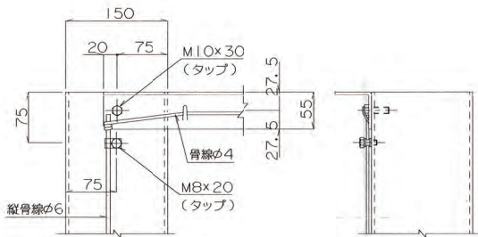
A'部詳細図 s=1/5
