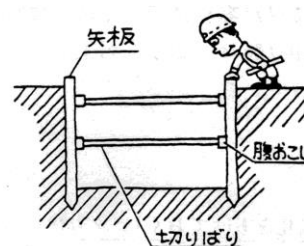
土留め工事
