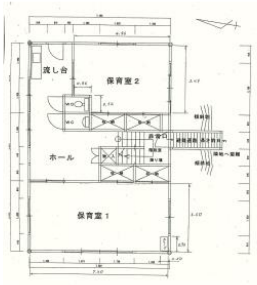
建物②2階
