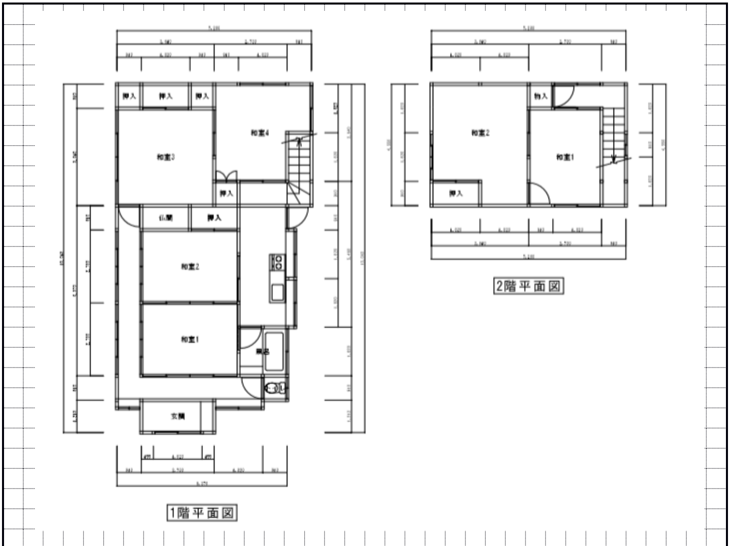
間取り図
