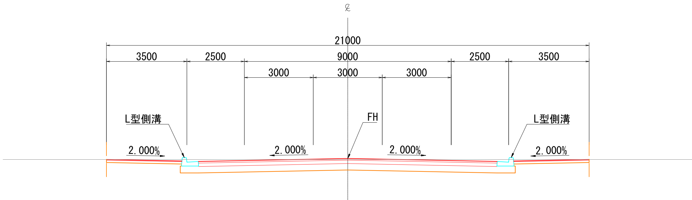
標準横断面図（交差点部）
