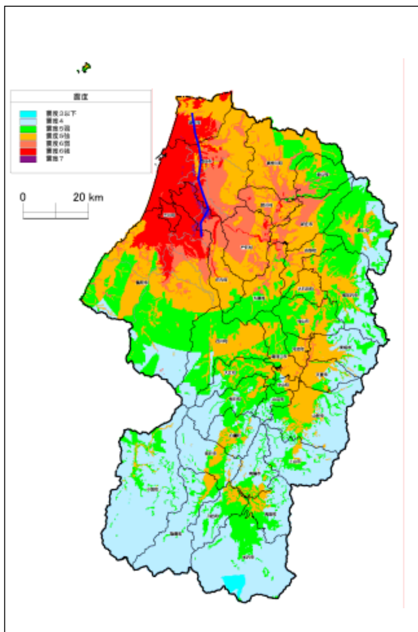
図 震度分布
