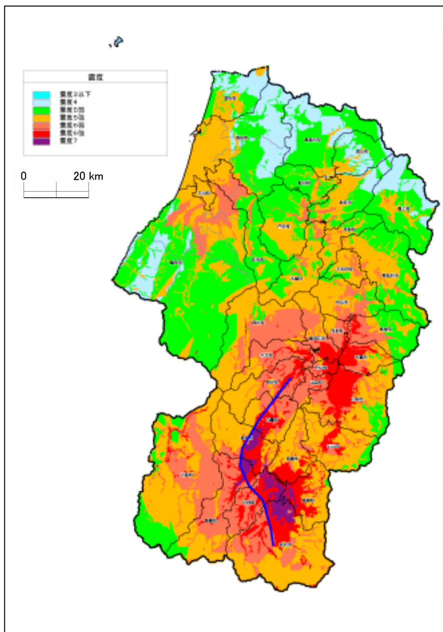
図 震度分布
